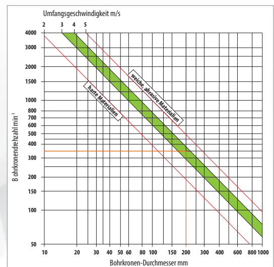
Korrekte Drehzahl Ihres Bohrmotors in Abhängigkeit vom Bohrkronendurchmesser und der Härte des zu bohrenden Materials.
